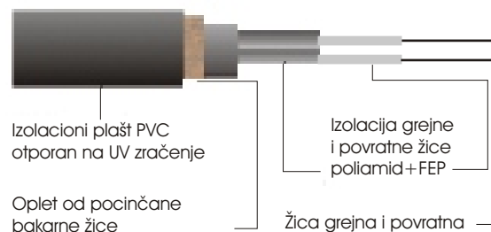
Poprečni presek žica SHTL 20 Jednostrano napajanje
