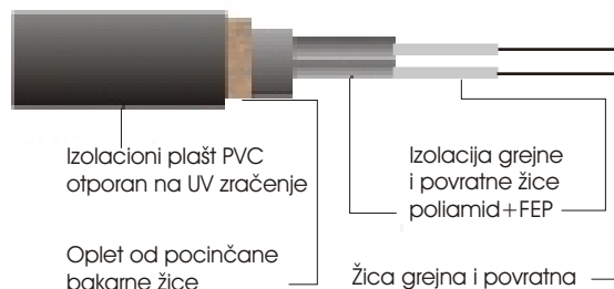
Poprečni presek žica SHTL 30 Jednostrano napajanje
